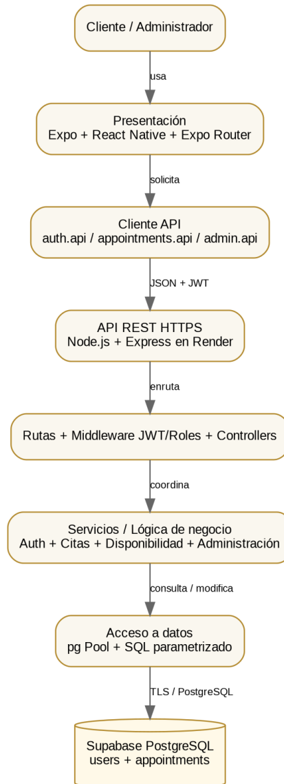
Arquitectura cliente-servidor de Barbería Cale v1.0.
